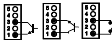
[20.2] Ejemplos de conexión. PNP, NPN o contacto libre. Sin tensión externa.
