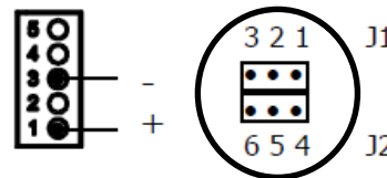
[20.3] Conexión con tensión externa. Colocar puente entre J1(2) y J2(5)
