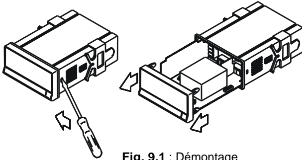
Fig. 9.1 : Démontage
