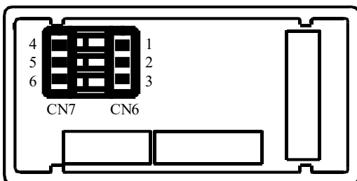
Vue postérieure instrument de base avec option sorties RELAIS / OPTOS
