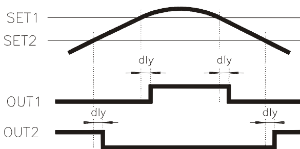
Fig. 1 Retard par temporisation (dly)
